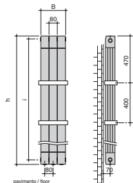
Modello 3 elementi con 2 barre Model 3 elements with 2 bars
