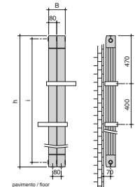
Modello 2 elementi con 2 barre Model 2 elements with 2 bars
