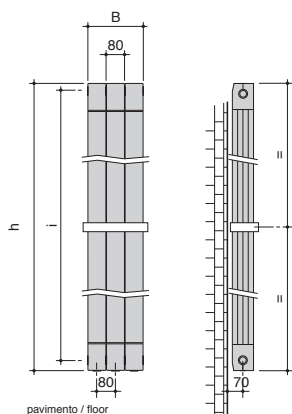
Modello 3 elementi con 1 barra Model 3 elements with 1 bar
